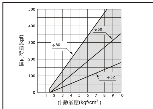
MSAR 常用荷重表
